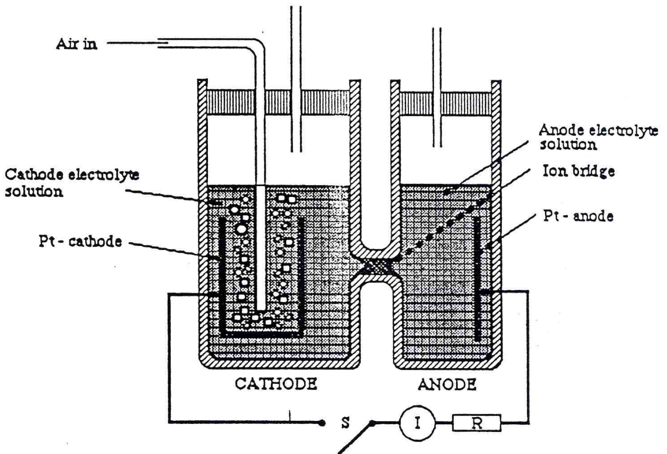
Schéma de la pile électrochimique.
