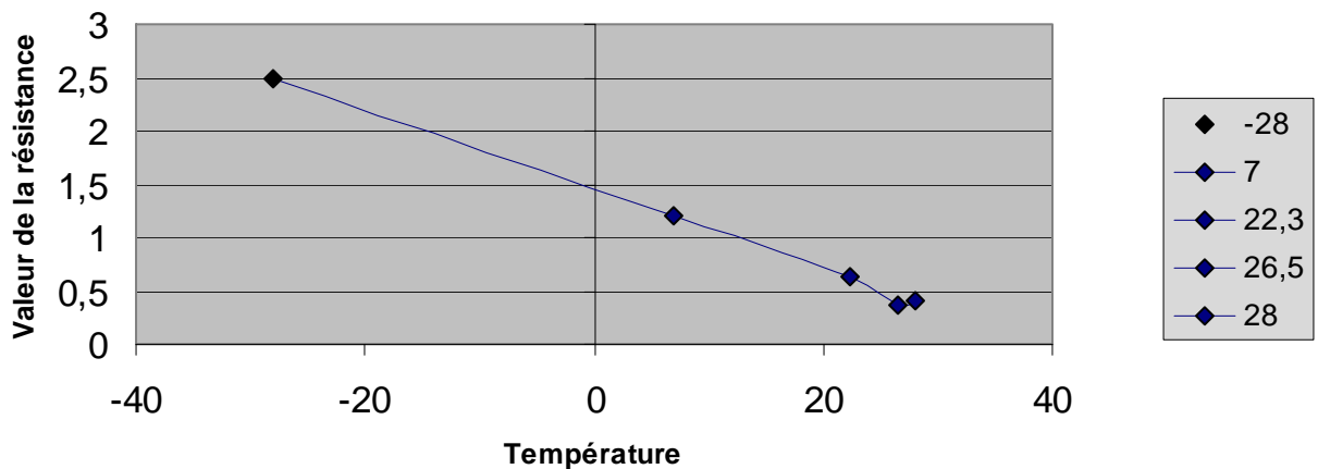
Valeur de la résistance de notre thermistance en fonction de la température
