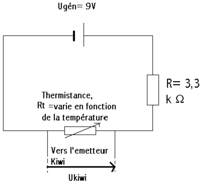
Schéma du circuit électrique de la thermistance.
